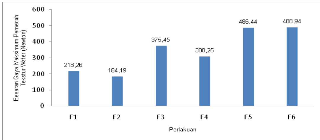
Gambar 3. Histogram besaran gaya maksimum pemecah pakan komplet berbentuk wafer dengan bahan utama jerami jagung
