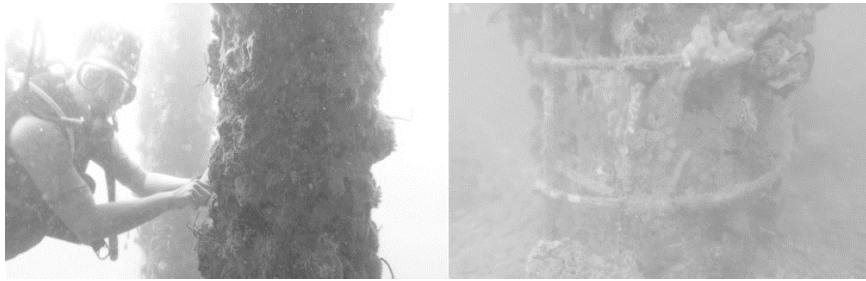
Gambar 2. Kondisi Struktur Bawah Dermaga (Tiang Pancang) yang mengalami kerusakan
