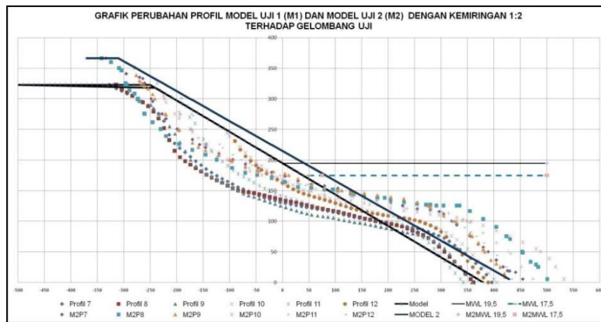
Gambar 2. Grafik Perubahan Profil Lereng Model Uji 1 (M1) dan Model Uji 2 (M2) dengan kemiringan 1:2
